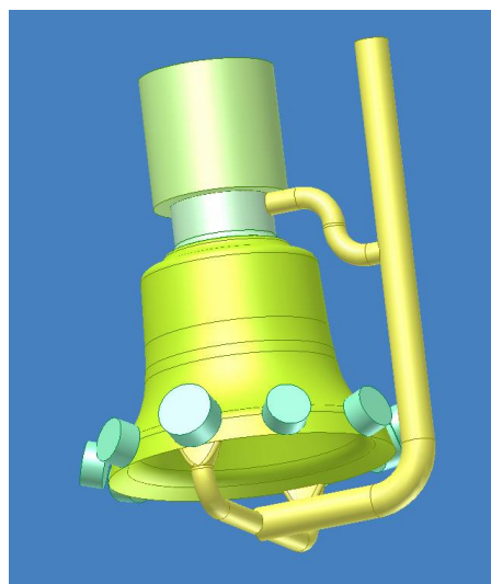
Obrázek 2: 3D model surového odlitku
