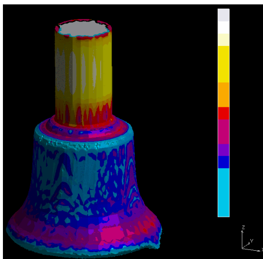
Obrázek 4: Simulace chlazení odlitku ve formě
