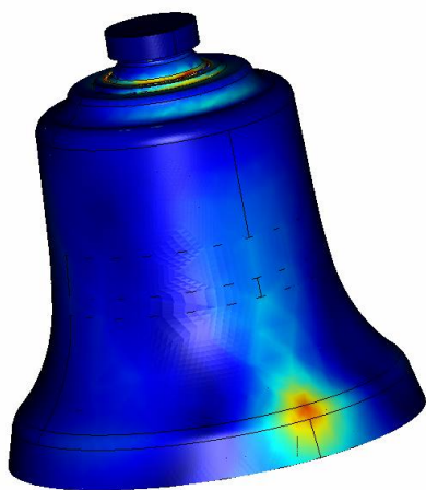
Obrázek 5: Napjatost ve zvonu
