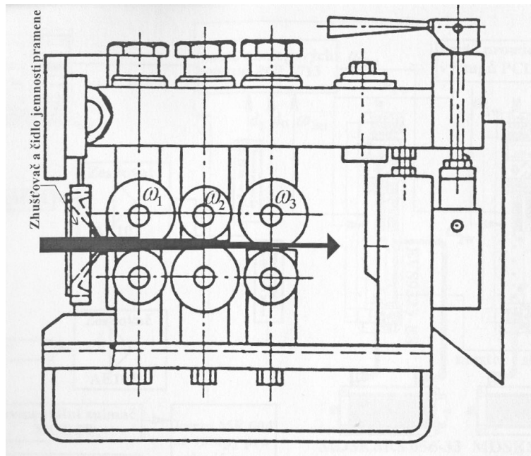
Obrázek 2: Průtažné ústrojí.
