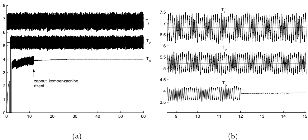
Obrázek 9: (a) Simulované časové průběhy jemností, (b) detail.
